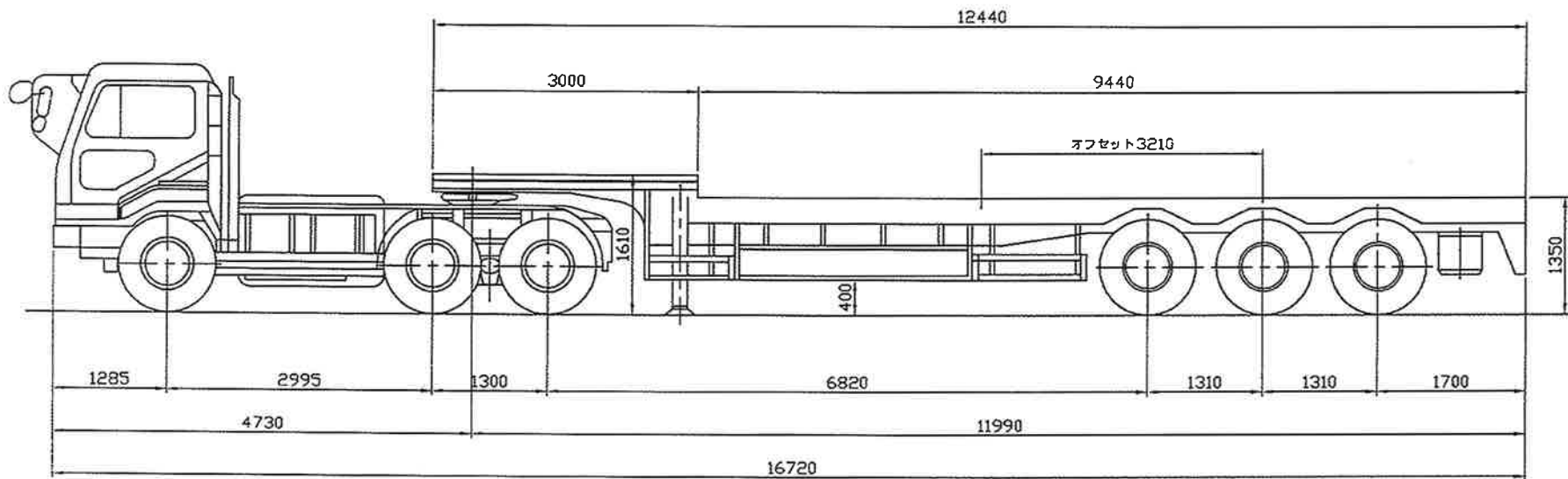
(ニッサンディーゼルトラクタ)
